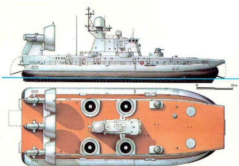
Рис. 3.18 – Малий десантний корабель на повітряній подушці “Зубр”
