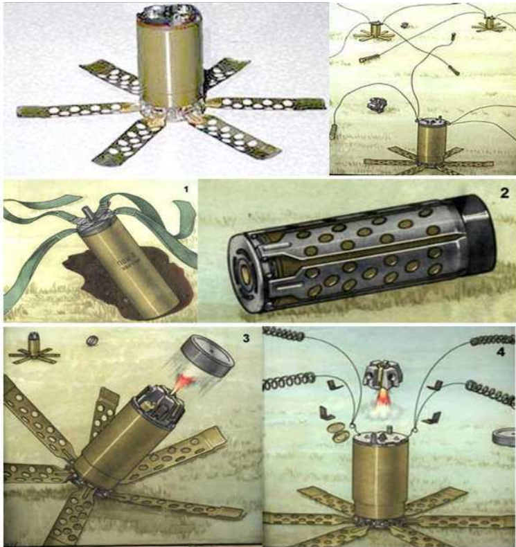
Рис. 1.171 – Протипіхотна фугасна міна дистанційного мінування таяжної дії ПОМ-2 та порядок встановлення на місцевості
