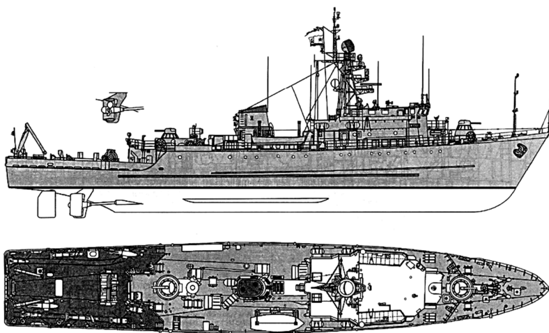
Рис. 3.25 – Морський тральщик проекту 266М
