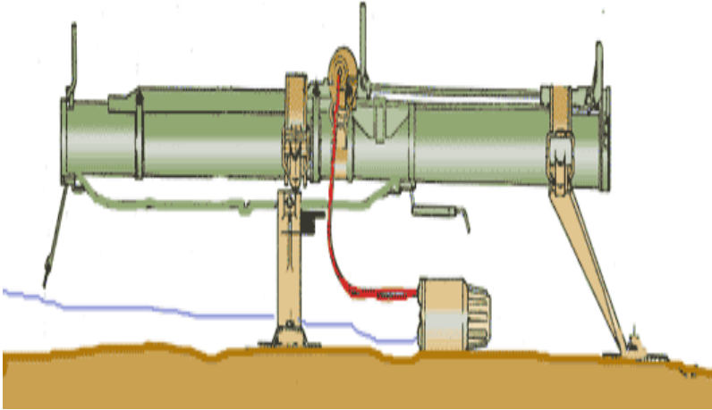
Рис. 1.175 –Протитанкова протибортова міна ТМ-73
