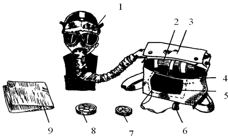
Рис. 1.197 – Ізолюючий дихальний апарат ИП-4М: 1) маска МИА-1; 2) регенеративний патрон РП-4; 3) торба; 4) каркас; 5) дихальний мішок; 6) пробка; 7) мембрани переговорного пристрою; 8) незапiтнiлi плiвки; 9) мiшок для зберiгання
