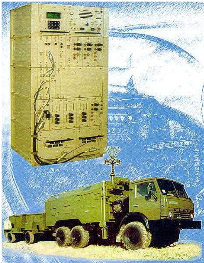
Рис. 2.107 – Радіостанція Р-997
