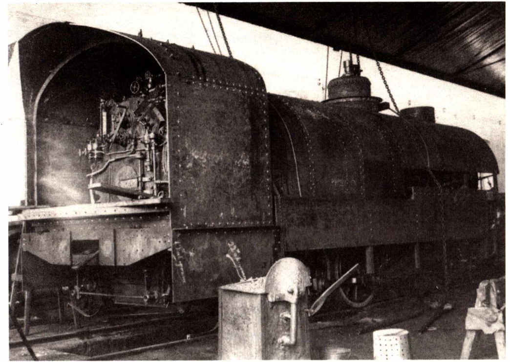
Будівництво панцирного потяга типу «Хунхуз» у майстернях Київського політехнічного інституту під час Першої світової війни.
