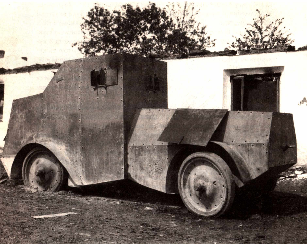
Панцирник, збудований за проектом Віктора Поплавка, літо 1917 р., вид збоку. Фото з колекції Олександра Пересацька
