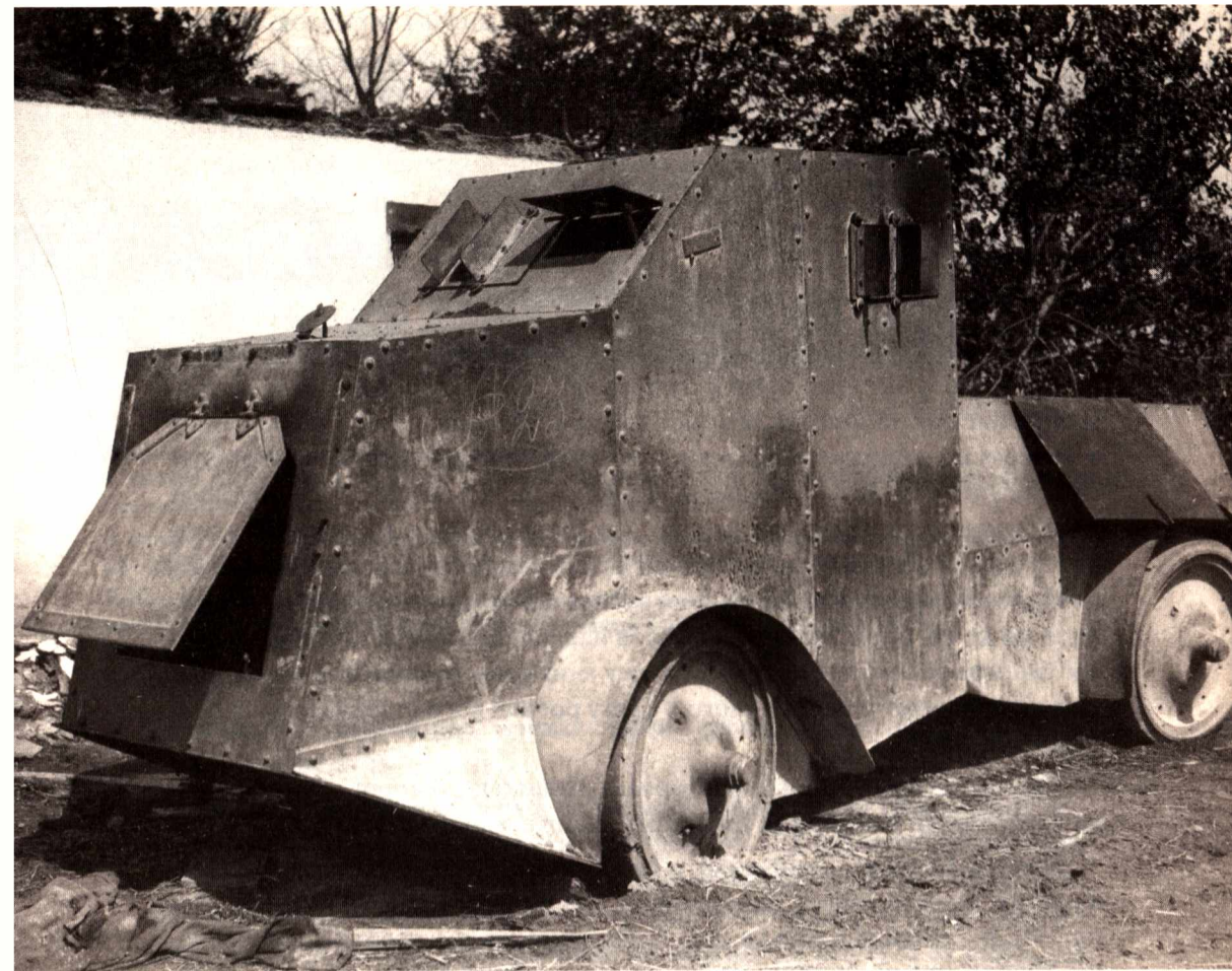
Панцирник, збудований за проектом Віктора Поплавка, літо 1917 р., вид спереду. Фото з колекції Олександра Пересацька
